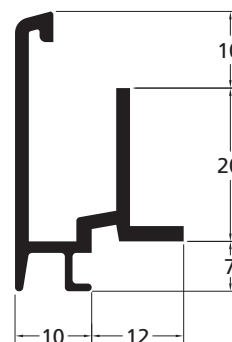
Artikelnummer 166450 (schaal 1:1)
